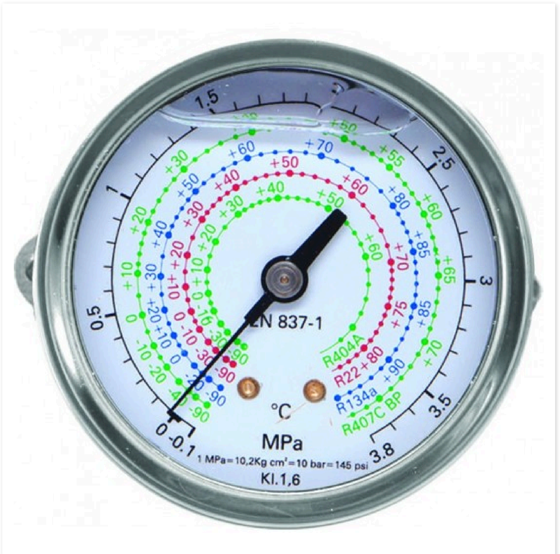
MANOMETRO GLICERINA IN ACCIAIO INOX CON STAFFA E VITI DI FISSAGGIO MAN-SAE-OIL-63-S1-H-P-I - R22-134-404-407
