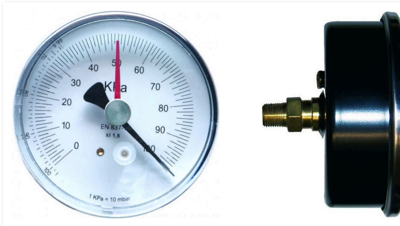
MANOMETRO PER VUOTO MAN-VUOTO-NPT-80-0-1000-P - 1/8" NPT - POSTERIORE CENTRALE
