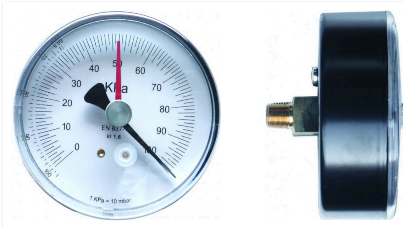
MANOMETRO PER VUOTO MAN-VUOTO-NPT-63-0-1000-P - 1/8" NPT - POSTERIORE CENTRALE
