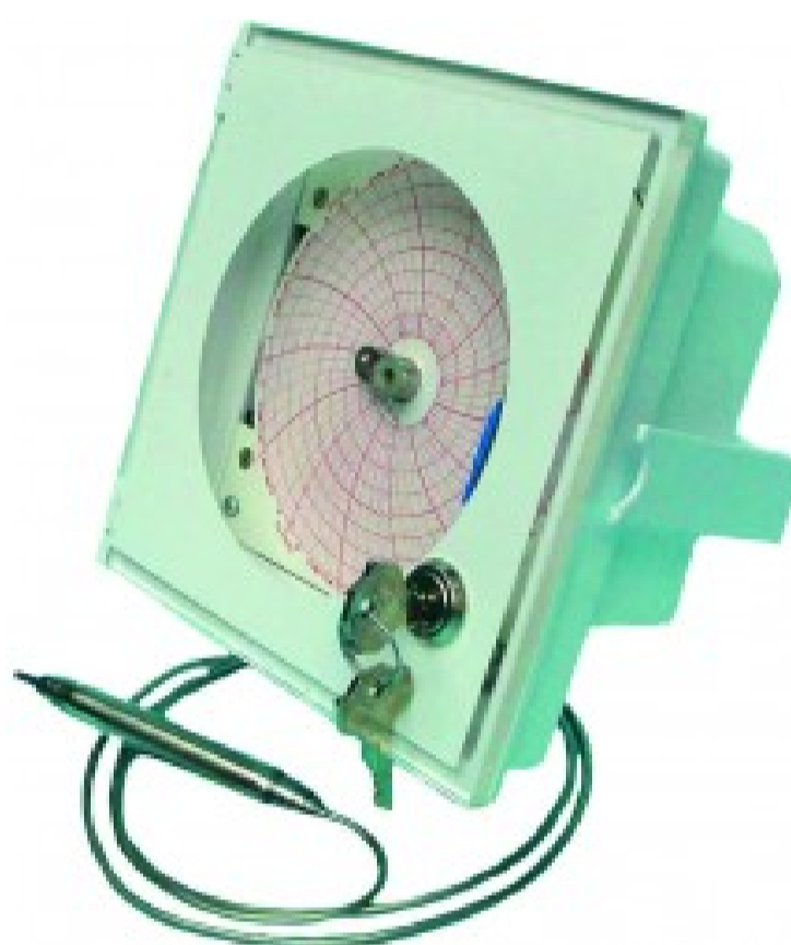
Termoregistratore grafico a gas inerte RTD-Q-35+15-JR - -35°C
