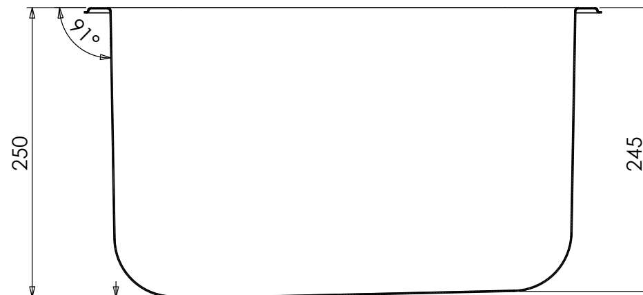
SEZIONE B-B
