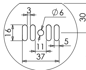
DETTAGLIO C
